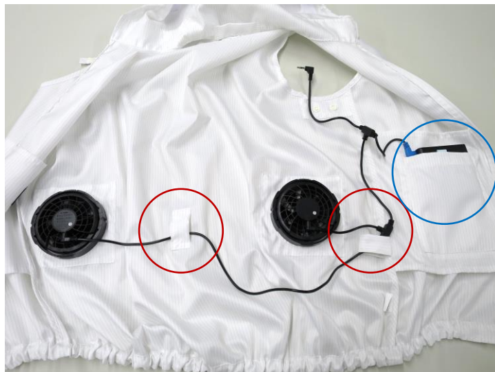
プラグ・ジャックの組み合わせ
